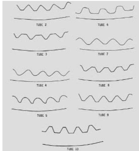
Fig. 11. Fin profiles for micro-fin tubes (Khanpara et al., 1986).
